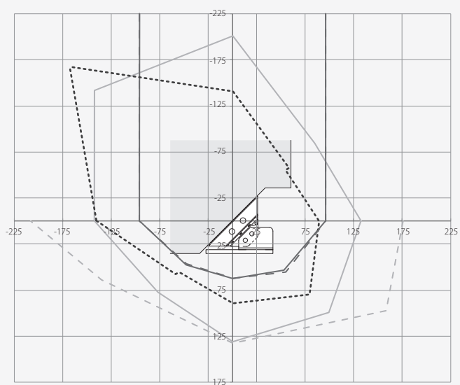
X-PLATE BMAXIL/R - Dominio de resistencia de proyecto
