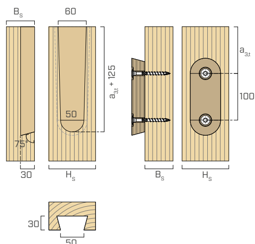
Ausfräsung
