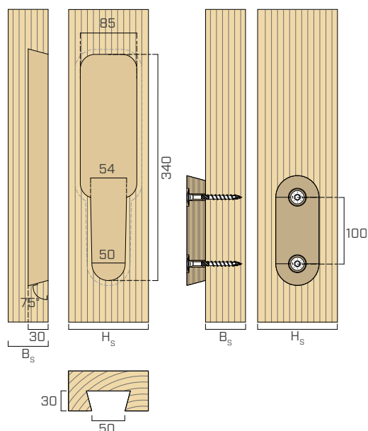
Ausfräsung
