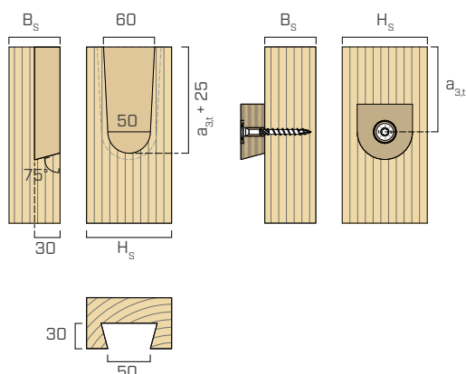
Ausfräsung
