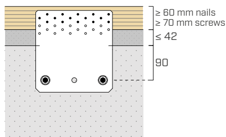
Teilaussnagelung 15 Befestigungen - C/GL
