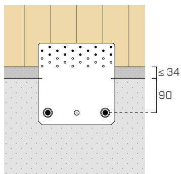
Teilaussnagelung 15 Befestigungen - BSP
