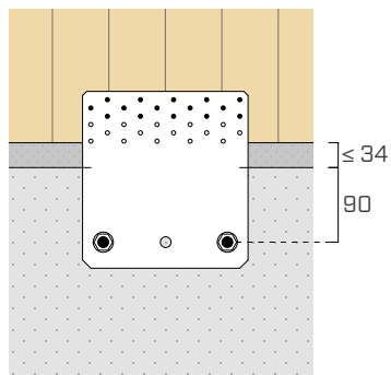
μερικο 15 μεσα συνδεση - CLT
