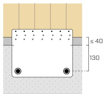
μερικο 7 μεσα συνδεση - CLT
