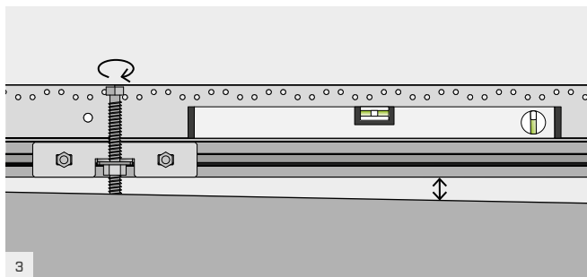
Uzdružno izravnavanje poluga ALU START.
