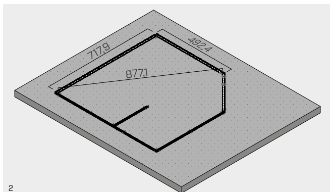
Definitivan tlocrt s provjerom duljina i dijagonala.
