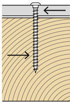
荷重と木目の角度 \alpha = 90^\circ
