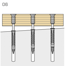
Regolare in maniera analoga le altre viti per livellare la struttura.
