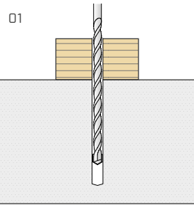
Forare gli elementi con un diametro dv = 8,0 mm.
