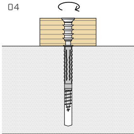
Fissare il listello avvitando la vite in maniera tale che la testa risulti a filo dell'elemento in legno.
