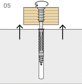
Allentare la vite in funzione della distanza desiderata.
