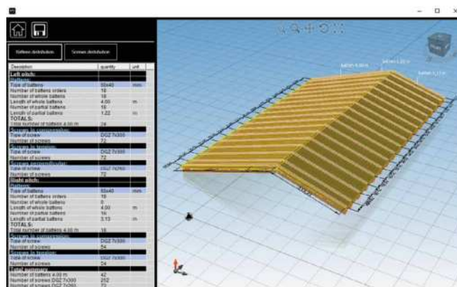
Aufmaß Dachlatten.
