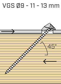
滑移连接 含 VGU 垫圈
