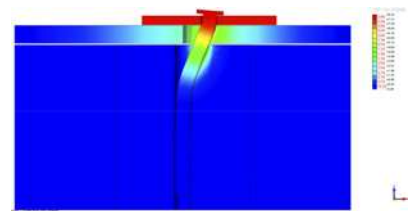
Écart Tx [mm] par écart induit de la plaque en acier égal à 8 mm
