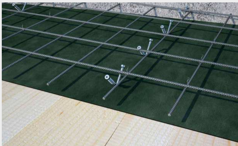
^ Fa-beton földem CLT panelen 45° - os csatlakozók szimpla sorozaton történő elhelyezésével.
