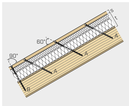
PEVNÁ ISOLÁCIA ZASTREŠENIA \sigma_{(10\%)} \geq 50 kPa (STN EN 826)
