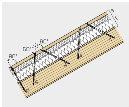
MÄKKÁ ISOLÁCIA ZASTREŠENIA \sigma_{(10\%)} < 50 kPa (STN EN 826)
