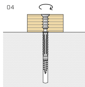
04 Upevnenie lišty zaskrutkovaním skrutky tak, že hlava je v jednej rovine s dreveným prvkom.
