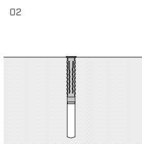
02 Vloženie nylonovej hmoždinky NDK GL do podpery.
