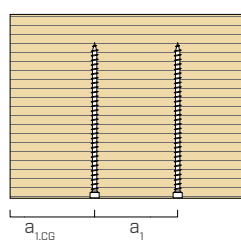
nárys
