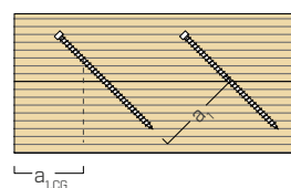
nárys
