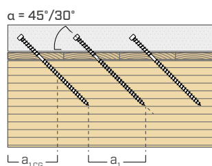
30°/45° yhdensuuntaiset
