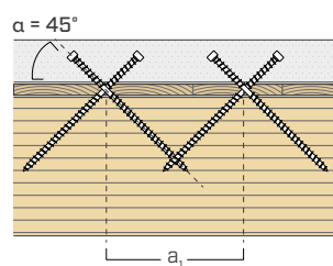
45° ristikkäiset
