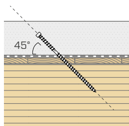
Asennus 45° äänieristyslevyllä.
