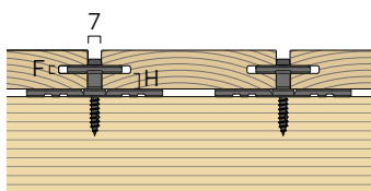
매립형 패스너
