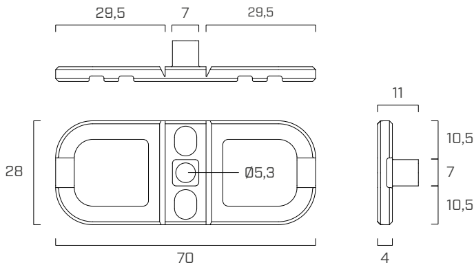
가시형 패스너
