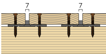
가시형 패스너
