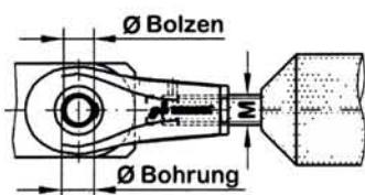
Druckstabanschluss aus Rundstab
