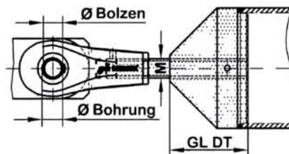
Druckstabanschluss zweiteilig mit Rohr
