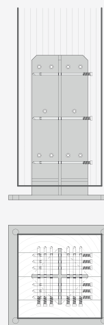
Prekryté spojenie na základe stĺpovej konzoly typu x10.
