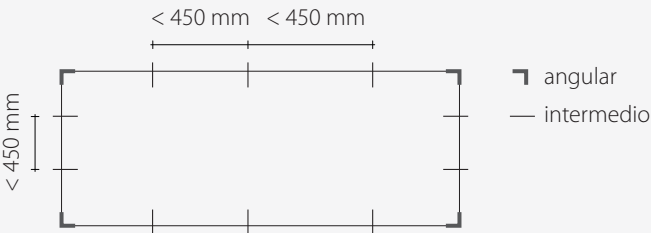
Distancia máxima para el posicionamiento correcto de los elementos de soporte
