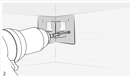
Fixação dos suportes com parafusos incluídos na embalagem.
