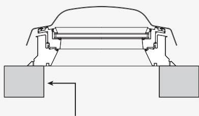
Aplicação do elemento de suporte angular/intermediário.
